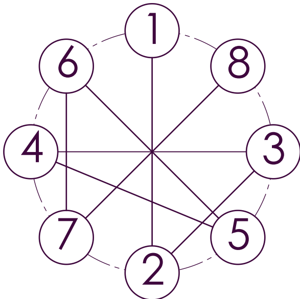
8 LUG PATTERN
