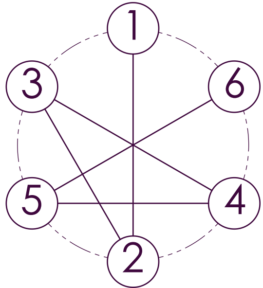
6 LUG PATTERN
